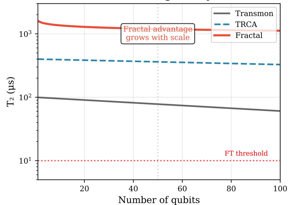
(d) Coherence Scaling with System Size
