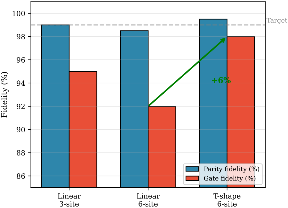
(d) Fidelity: Linear vs T-Junction
