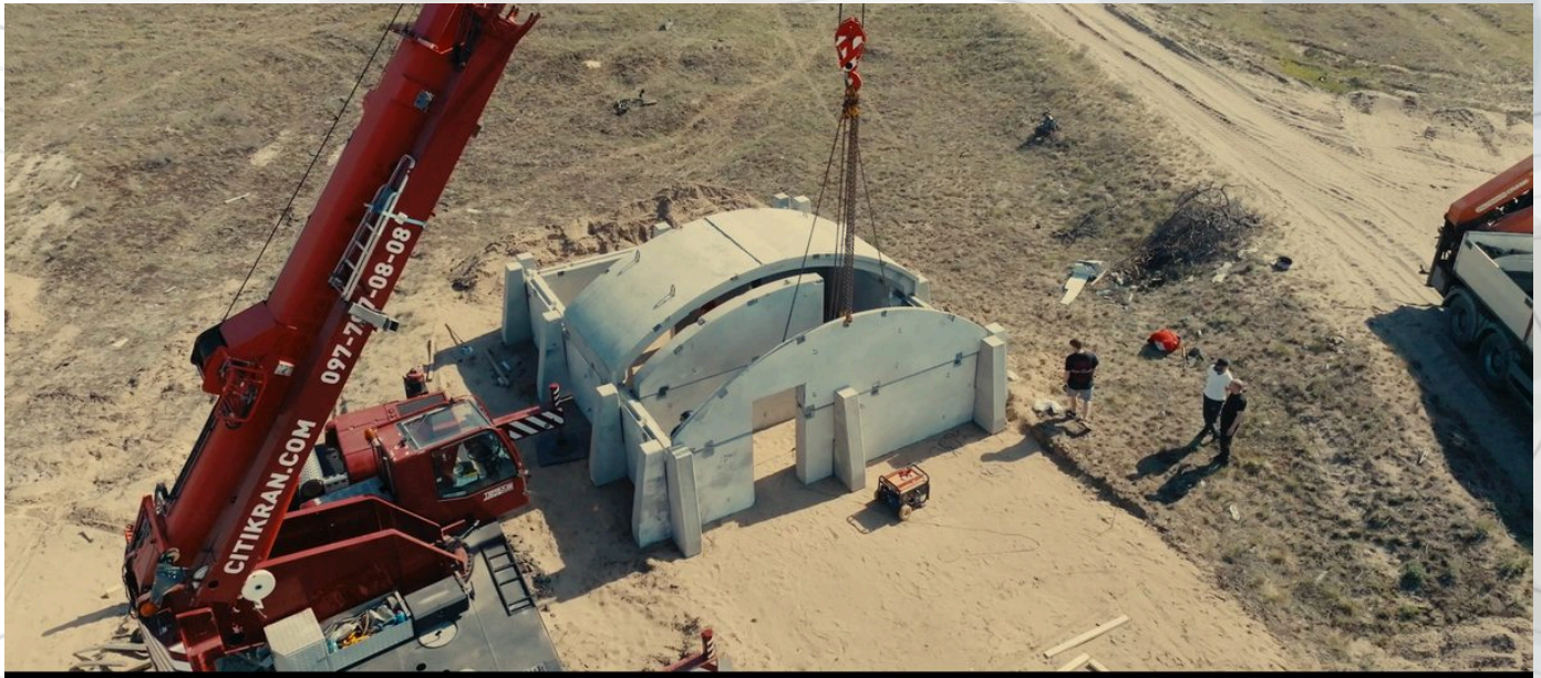
МОНТАЖ НАЗЕМНОГО МОДУЛЯ
