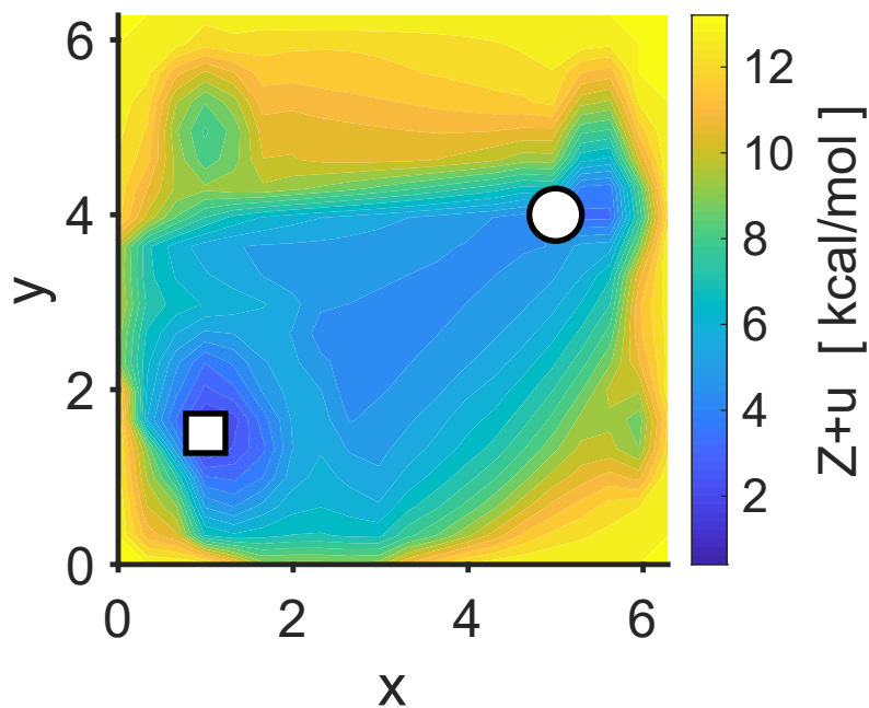
MFPT-opt U_{\max}=6 k_B T
