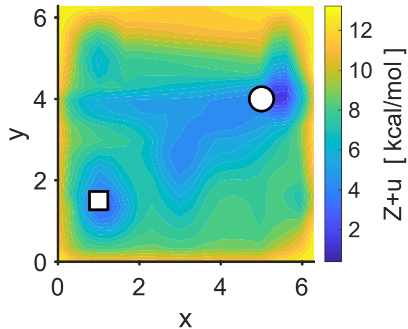
MFPT-opt U_{\max}=6 k_B T
