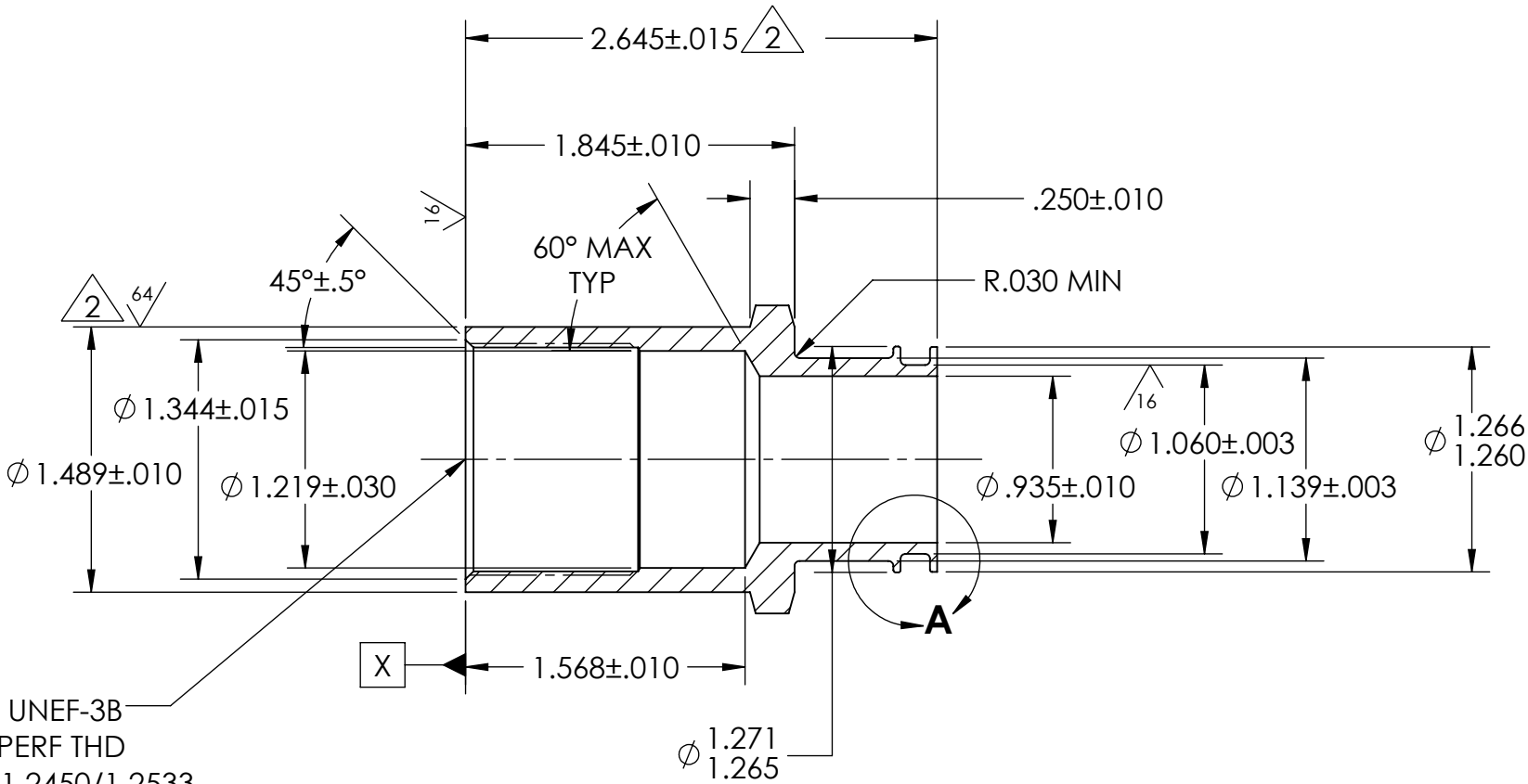
SECTION A-A
