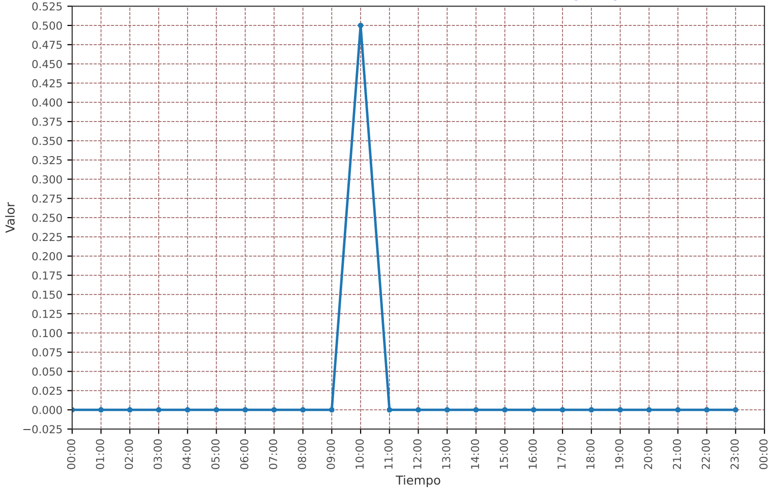
VOLCAN COTOPAXI - SERIE TEMPORAL (mm)
