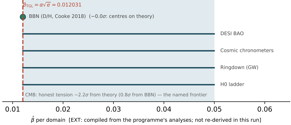
Figura 2: A convergência de \beta_{\text{TGL}} = \alpha\sqrt{e} por domínio. BBN centra na teoria ( -0,0\sigma ); os demais domínios caem na banda 0,012–0,050; a tensão CMB ( \sim 2,2\sigma ) é a fronteira honesta. [EXT: compilação das análises do programa (tgl_paper_unified.py), não re-derivada nesta rodada; a linha \beta_{\text{TGL}} é recomputada ao vivo.]
