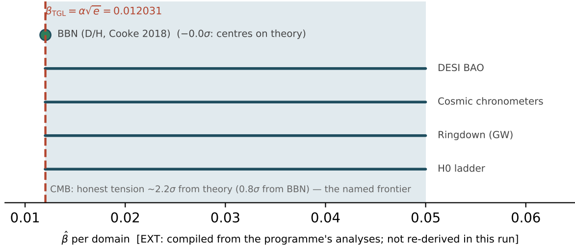
Figura 2: A convergência de \beta_{\text{TGL}} = \alpha\sqrt{e} por domínio. BBN centra na teoria (-0,0\sigma) ; os demais domínios caem na banda 0,012–0,050; a tensão CMB ( \sim 2,2\sigma ) é a fronteira honesta. [EXT: compilação das análises do programa (tgl_paper_unified.py), não re-derivada nesta rodada; a linha \beta_{\text{TGL}} é recomputada ao vivo.]
