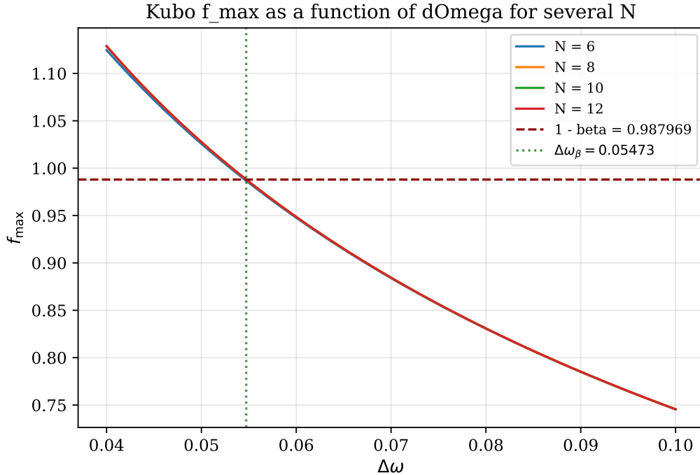
Figura 14: Bisseccão de Kubo: f_{\text{max}}(\Delta\omega) atravessa 1 - \beta_{\text{TGL}} exatamente em \Delta\omega_\beta = 0,054726411295 .
