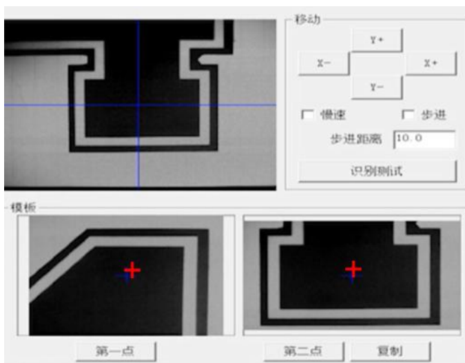
多点定位展示
