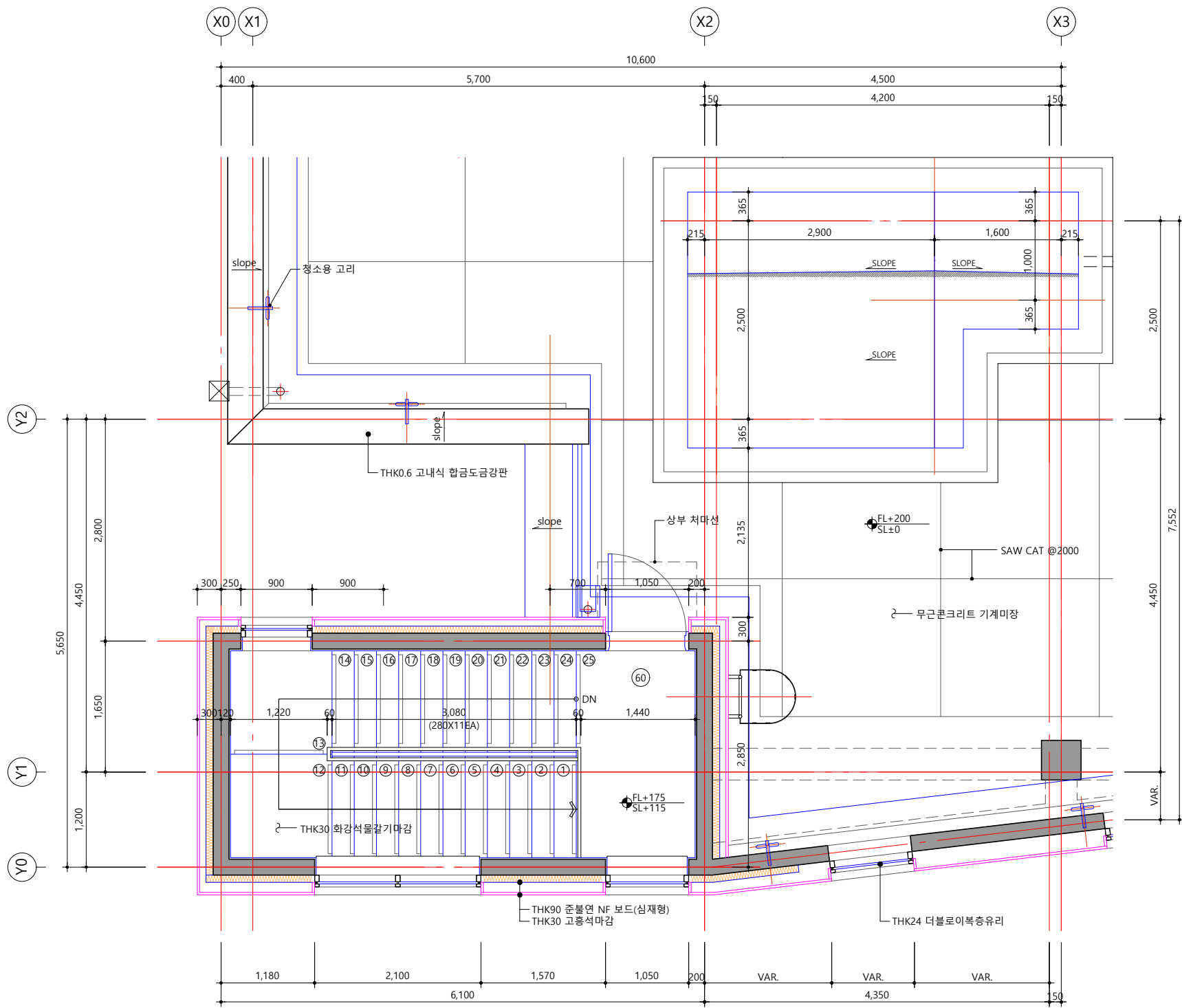
1 지붕 계단실 확대평면도 SCALE: 1 / 60
