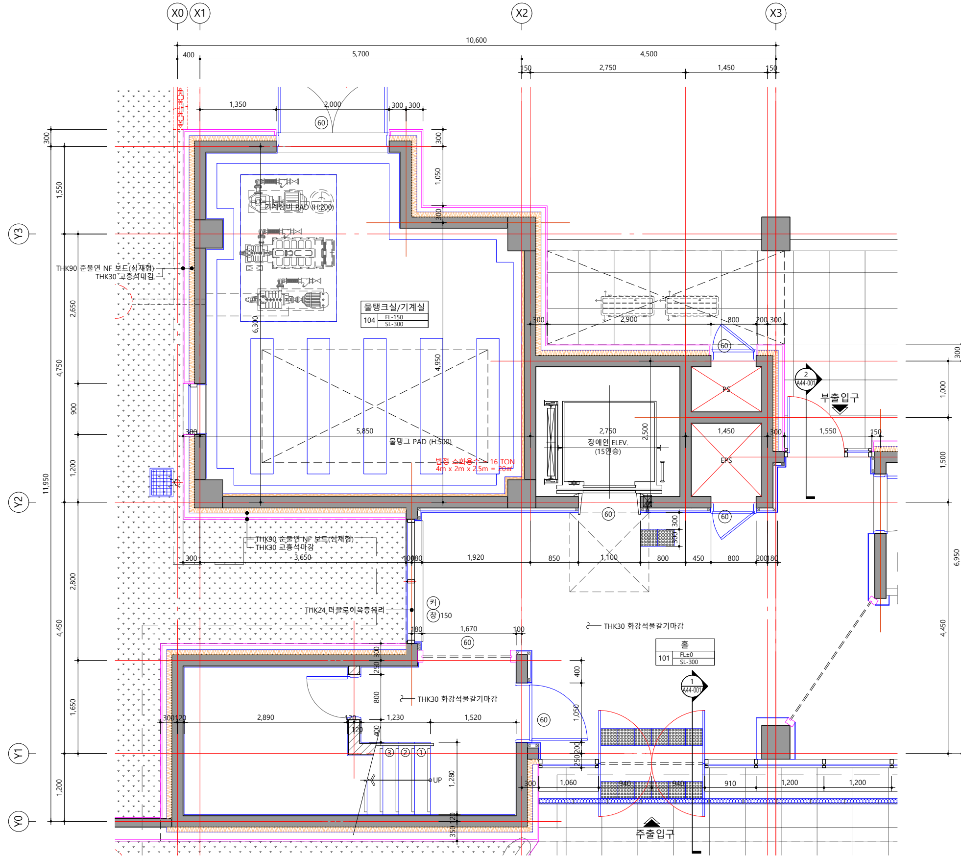
1층 계단실 확대평면도 SCALE: 1/60
