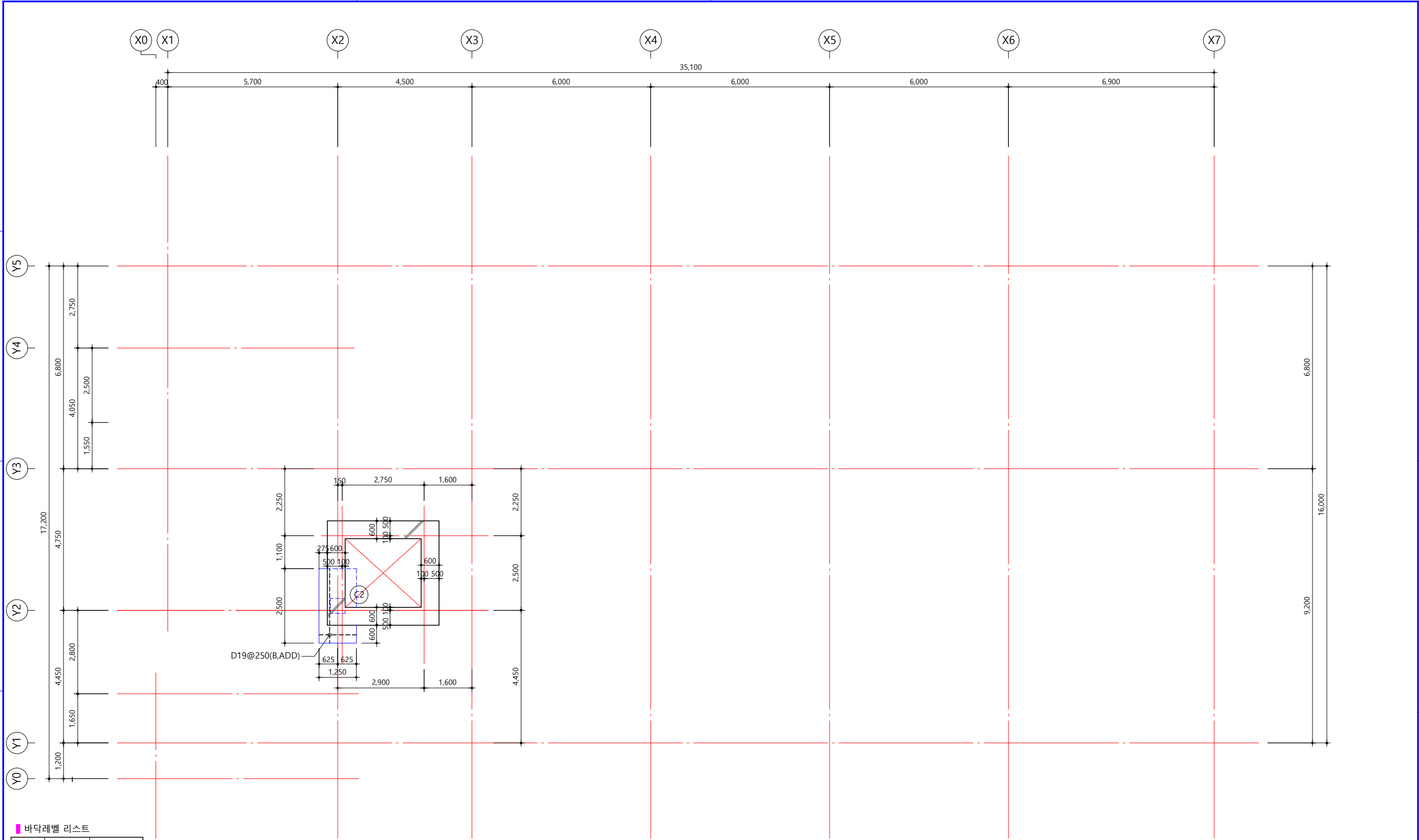
PIT 바닥 구조 평면도 SCALE : 1 / 120
