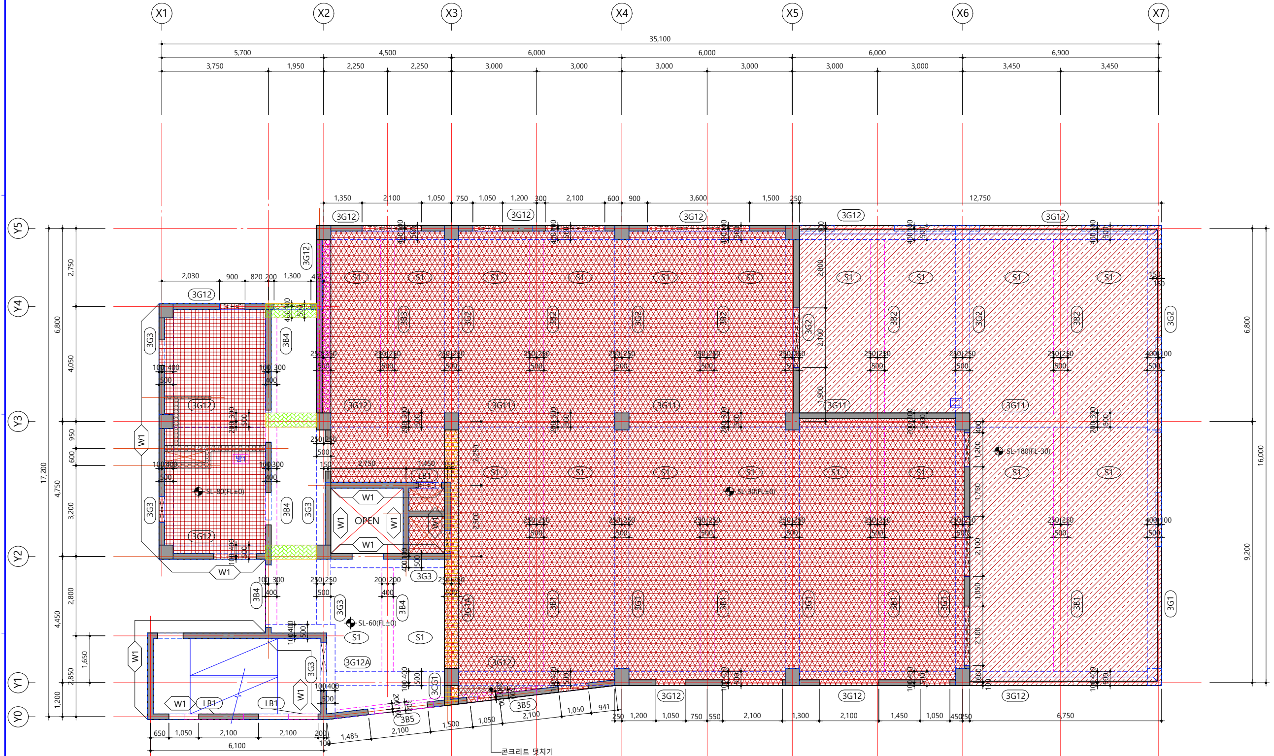
3층 바닥 구조 평면도 SCALE : 1 / 120
