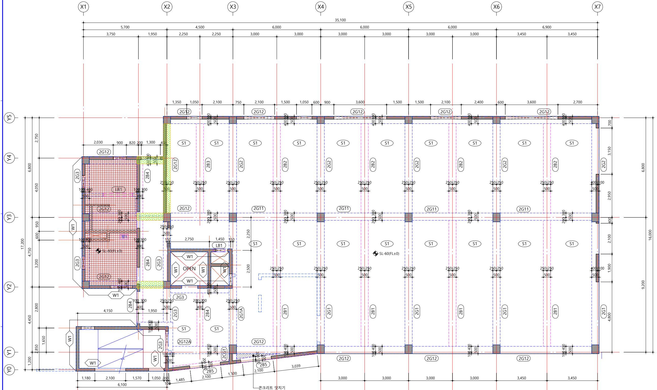
2층 바닥 구조 평면도 SCALE : 1 / 120
