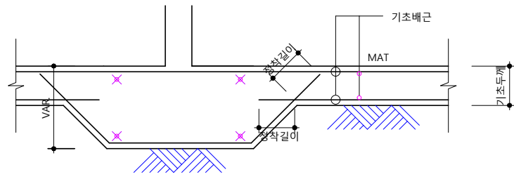
기초 하부보강 단면 상세
