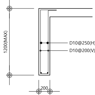
수벽 배근상세 (Thk. 200)
