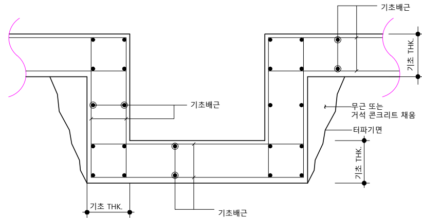
3 | ELEV. PIT 기초 단차부 배근 상세
