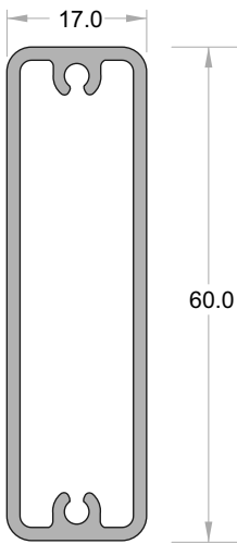
INFILL 60mm SLAT JVB/019/5.3
