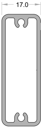
INFILL 49mm SLAT JVB/018/5.35
