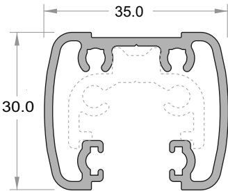
BOTTOM RAIL JVB/022/5.8w
