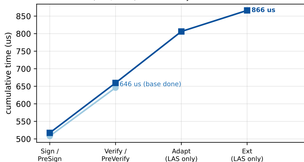
L5 (n=8, ell=7) — full LAS cycle +34.1% vs base
