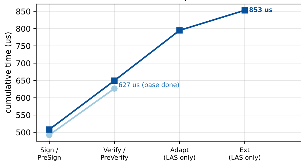
L5 (n=8, ell=7) — full LAS cycle +36.1% vs base
