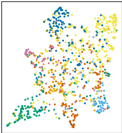
MLP
