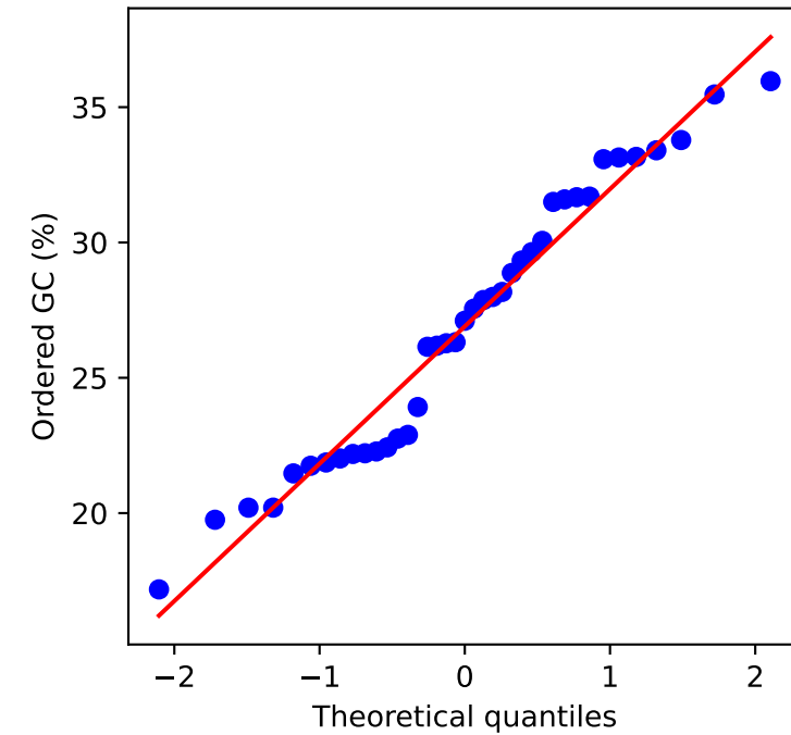
Dictyostelium discoideum
