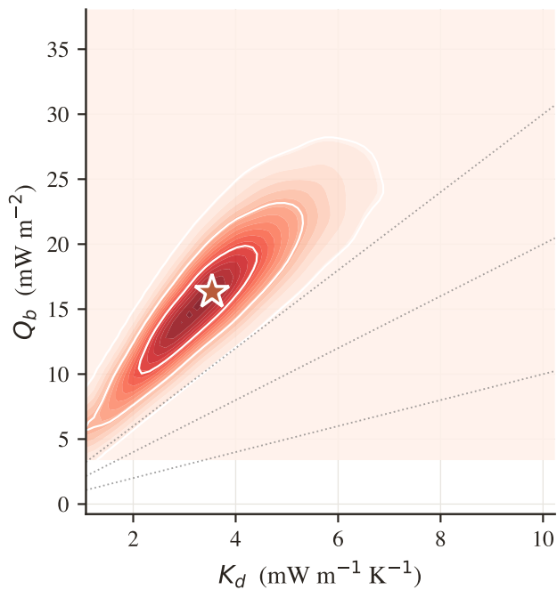
(a) Apollo 15 — joint posterior
