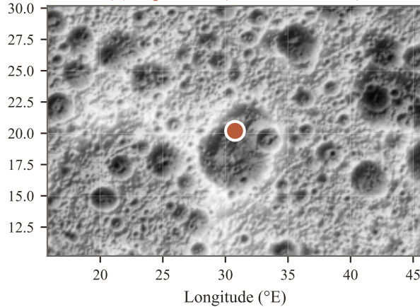
(d) Apollo 17 ( 20.2^{\circ} N, 30.8^{\circ} E)
