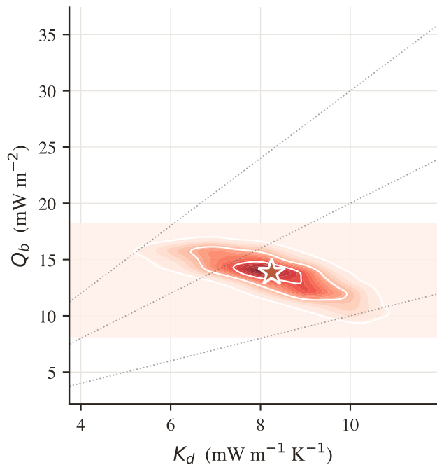
(b) Apollo 17 — joint posterior
