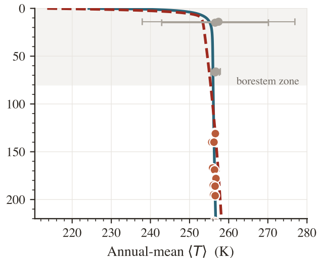
(d) Apollo 17 — deep-sensor zoom
