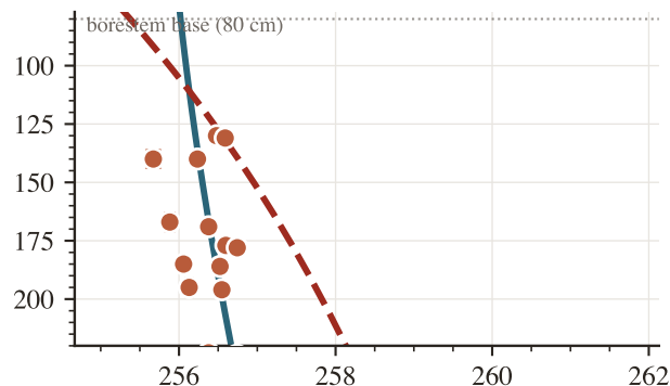
(d) Apollo 17 — deep-sensor zoom
