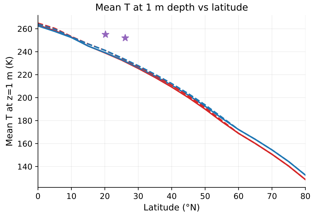
Mean T vs latitude — Fig 7 of Martinez & Siegler (2021)
