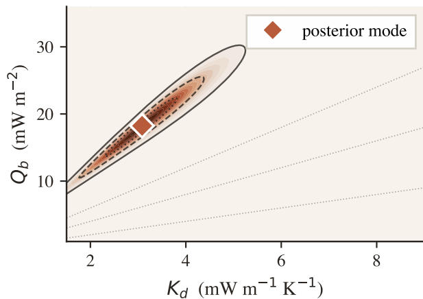
(a) A15 joint posterior
