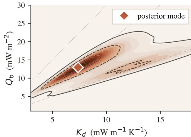
(b) A17 joint posterior
