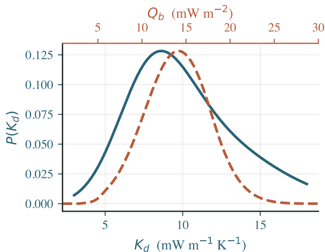
(d) A17 marginal posteriors
