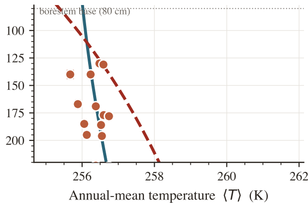
(d) Apollo 17 — deep-sensor zoom
