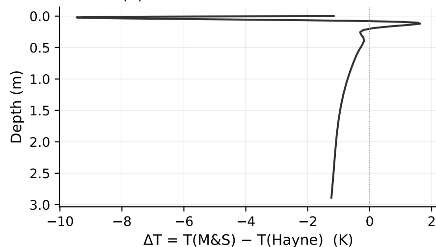
(d) Subsurface \Delta T at solar noon
