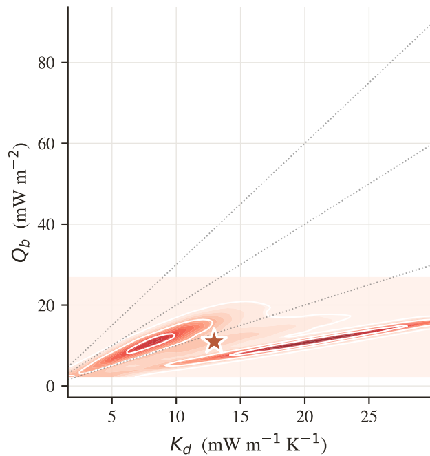
(b) Apollo 17 — joint posterior
