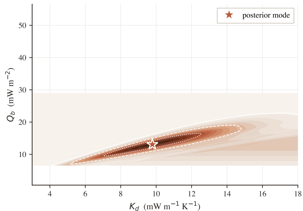
(b) A17 joint posterior
