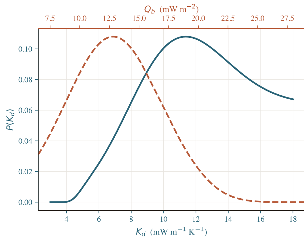
(d) A17 marginal posteriors
