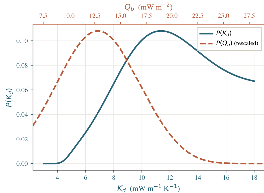
(d) A17 marginal posteriors
