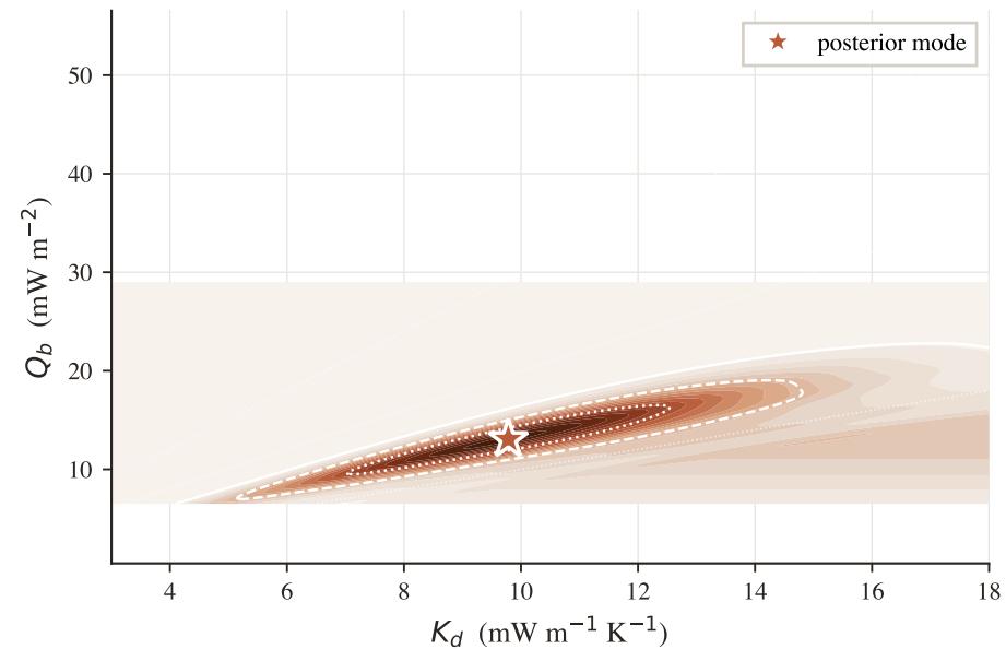
(d) A17 marginal posteriors
