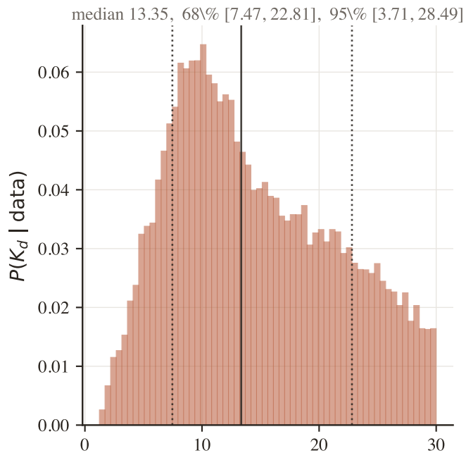
(d) Apollo 17 — marginal P(K_d)
