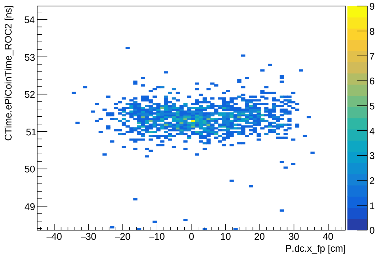
Phase 1 run 24041: CTime (ROC2) vs SHMS xfp
