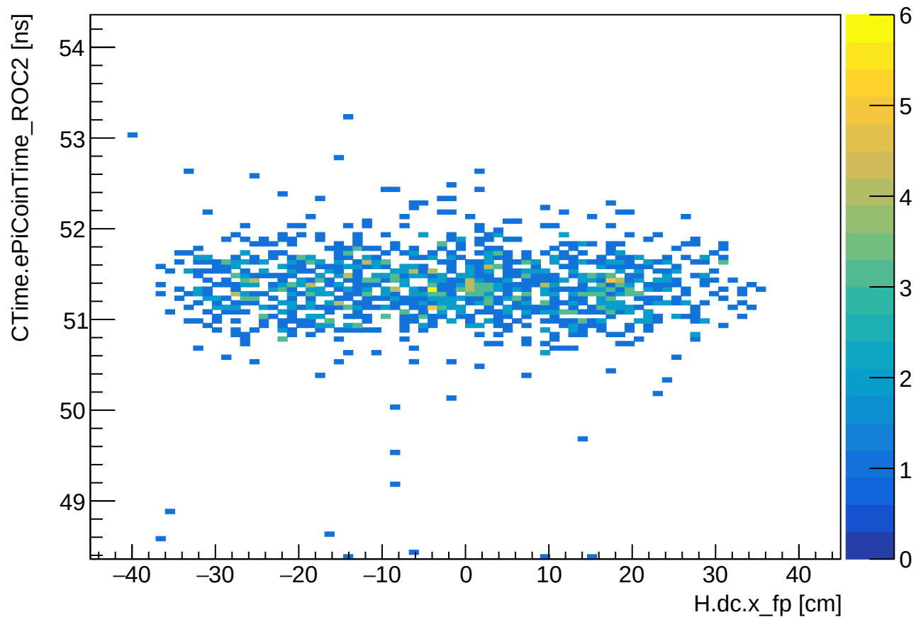
Phase 1 run 24041: CTime (ROC2) vs HMS xfp
