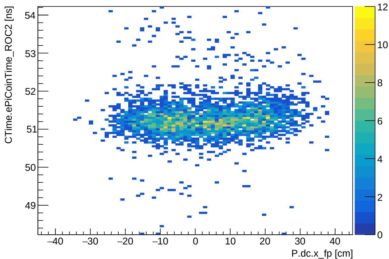
Phase 1 run 24647: CTime (ROC2) vs SHMS xfp
