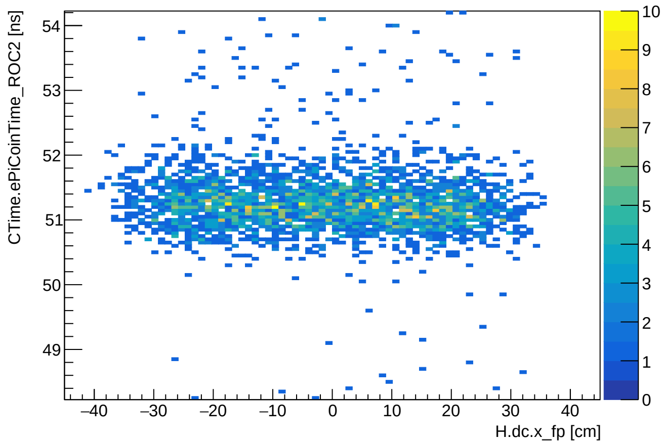
Phase 1 run 24621: CTime (ROC2) vs HMS xfp
