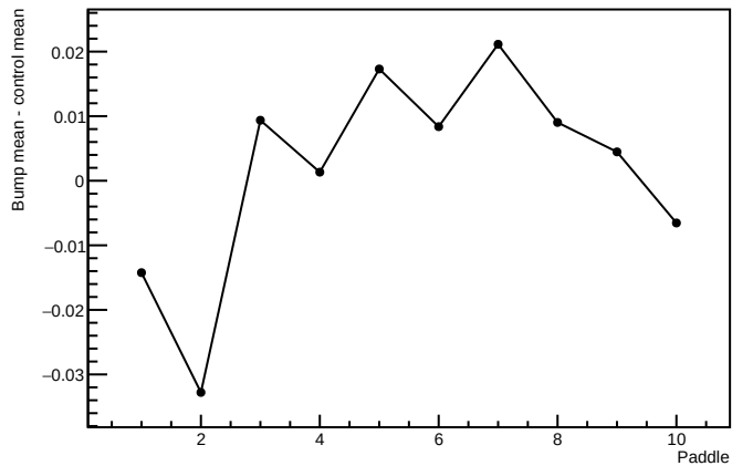
HMS 1y beta displacement
