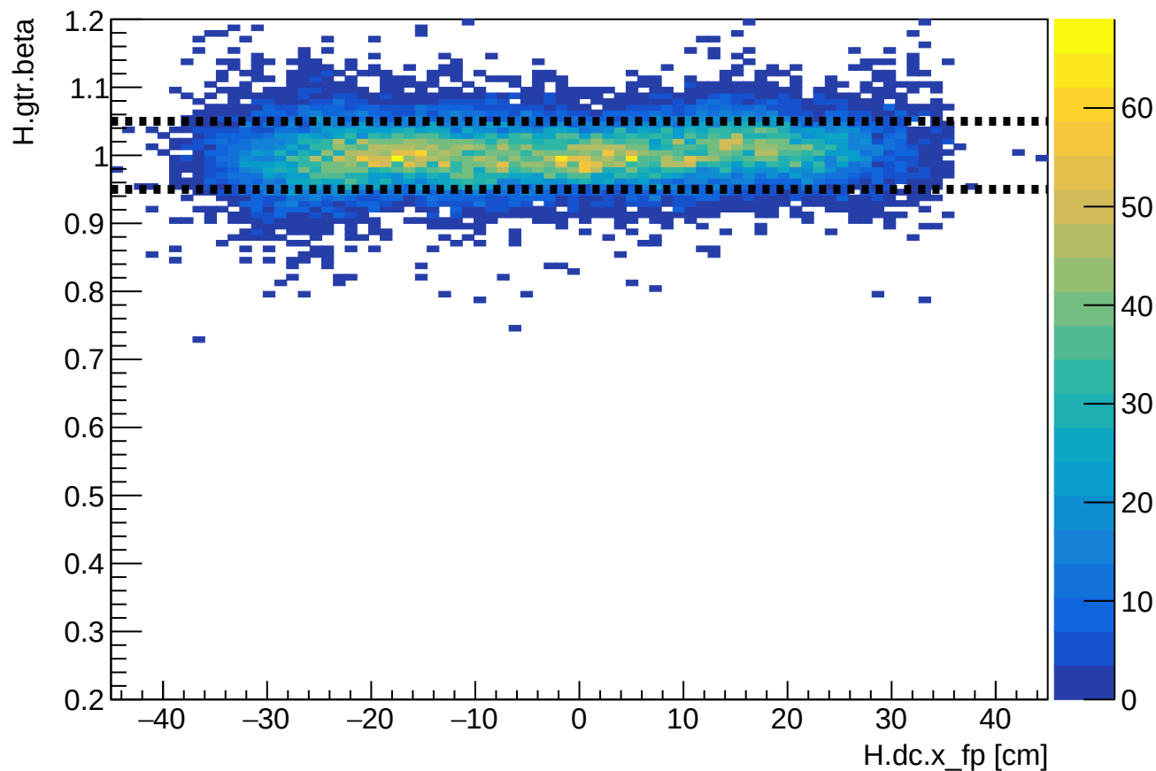
Phase 2 run 27264: HMS beta vs HMS xfp
