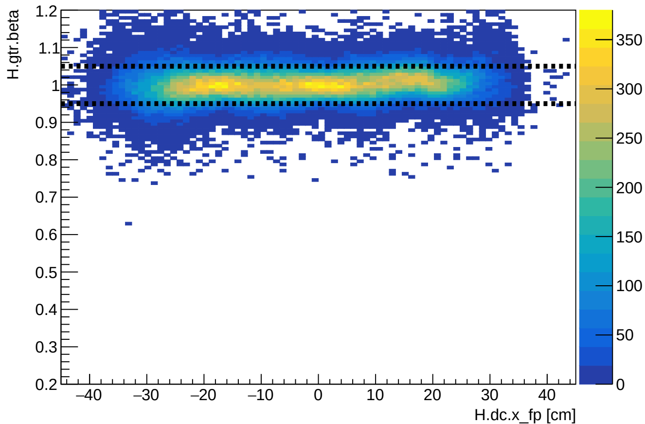
Phase 2 run 27262: HMS beta vs HMS xfp
