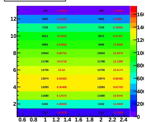
Preshower (Layer1)
