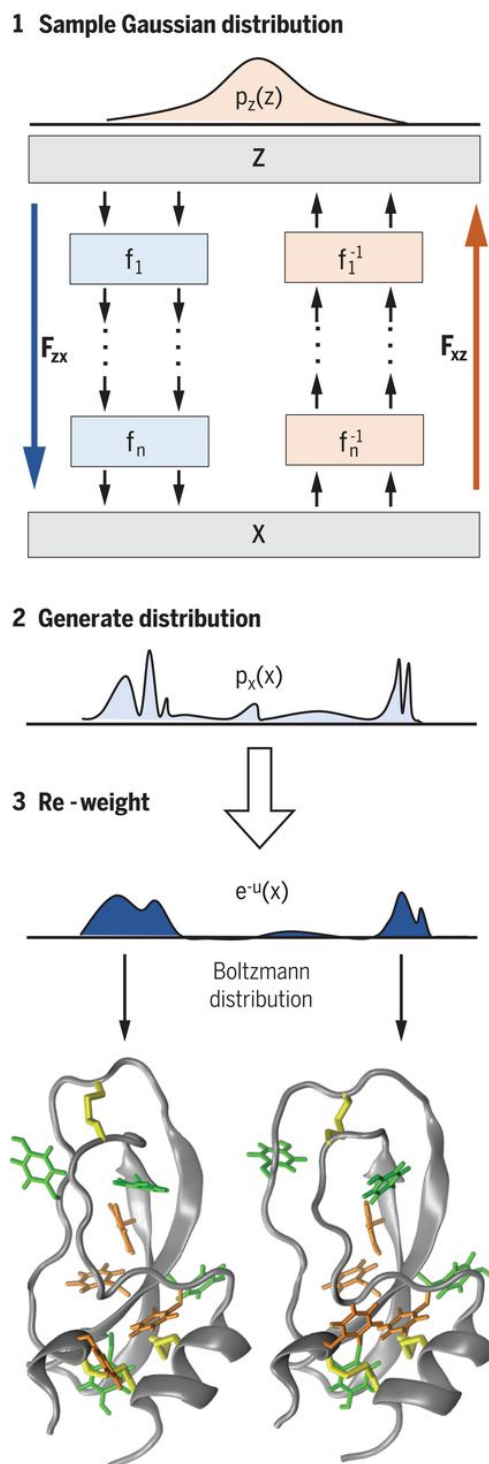
Figura 3.6: Boltzmann Generator: utilizza NF e Re-weighting per campionare la distribuzione di Boltzmann. Nella figura si mostrano i passi di questo metodo e due configurazioni di una proteina rappresentati due modi distinti della distribuzione target.
