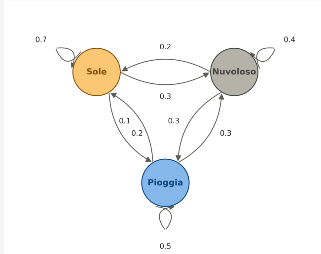
Figura 2.2: Diagramma degli stati e delle probabilità di transizione per la catena di Markov meteo a tre stati.
