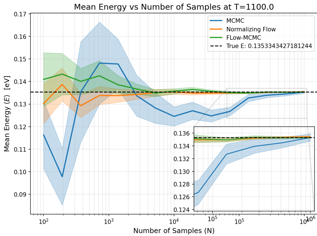
Figura 4.12: Energia media stimata da MCMC, NF e Flow-MCMC in funzione del numero di campioni N , per D = 3 a tre diverse temperature T = 100, 600, 1100 \text{ K} . La linea tratteggiata indica il valore di riferimento.
