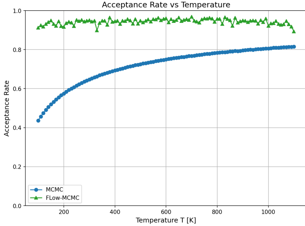
Figura 4.8: Tasso di accettazione di MCMC e Flow-MCMC in funzione della temperatura, a dimensione fissata D = 3 .
