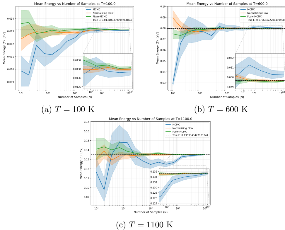
Figura 4.12: Energia media stimata da MCMC, NF e Flow-MCMC in funzione del numero di campioni N , per D = 3 a tre diverse temperature. La linea tratteggiata indica il valore di riferimento.
