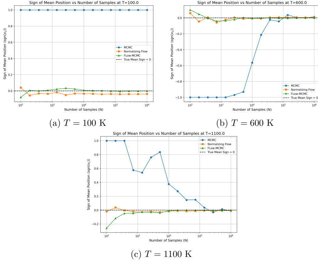
Figura 4.13: Segno medio \langle \text{sgn}(x_1) \rangle stimato da MCMC, NF e Flow-MCMC in funzione del numero di campioni N , per D = 3 a tre diverse temperature. Il valore teorico atteso è zero per ogni T .
