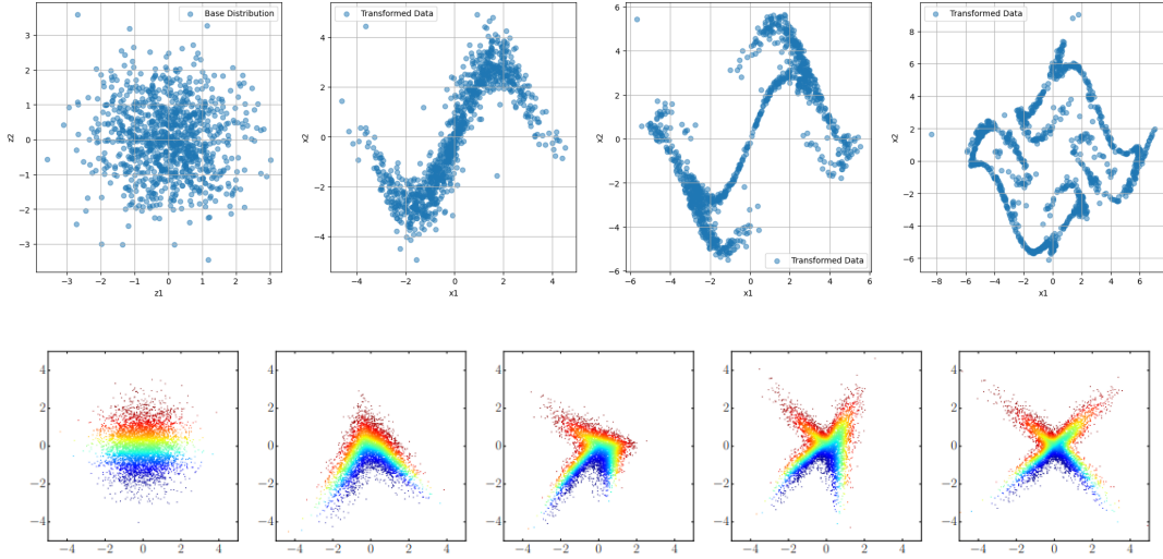
Figura 3.1: Esempi dell'effetto della composizione di trasformazioni per creare flow espressivi. In entrambe le immagini si campiona una distribuzione di base gaussiana e si applica progressivamente una sequenza di trasformazioni T_k , ottenendo distribuzioni qualitativamente molto diverse dalla base.
