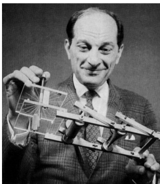
(a) Stanisław Ulam e il FERMIAC.
