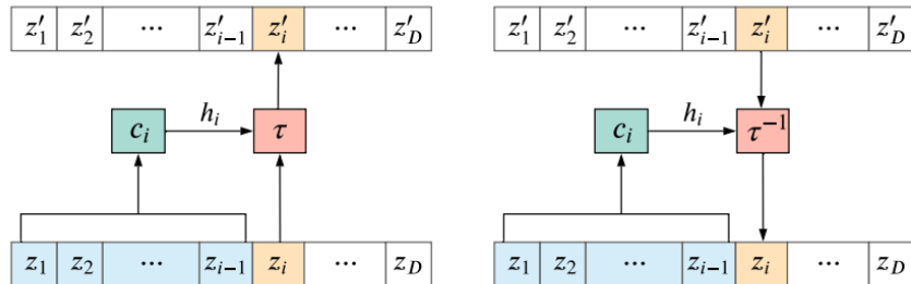
Figura 3.3: Rappresentazione grafica di un T_k autoregressive flow composto dal condizionatore c_i e dal trasformatore \tau . A sinistra la trasformazione e a destra la sua inversa.
