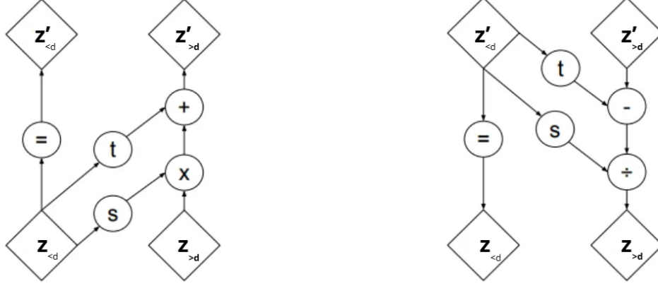
Figura 3.4: Rappresentazione grafica di un T_k per una Real NVP. Possiamo vedere la suddivisione del vettore \mathbf{z} e il calcolo di s e t rispettivamente i fattori di scaling e translation. A sinistra la trasformazione e a destra la sua inversa.
