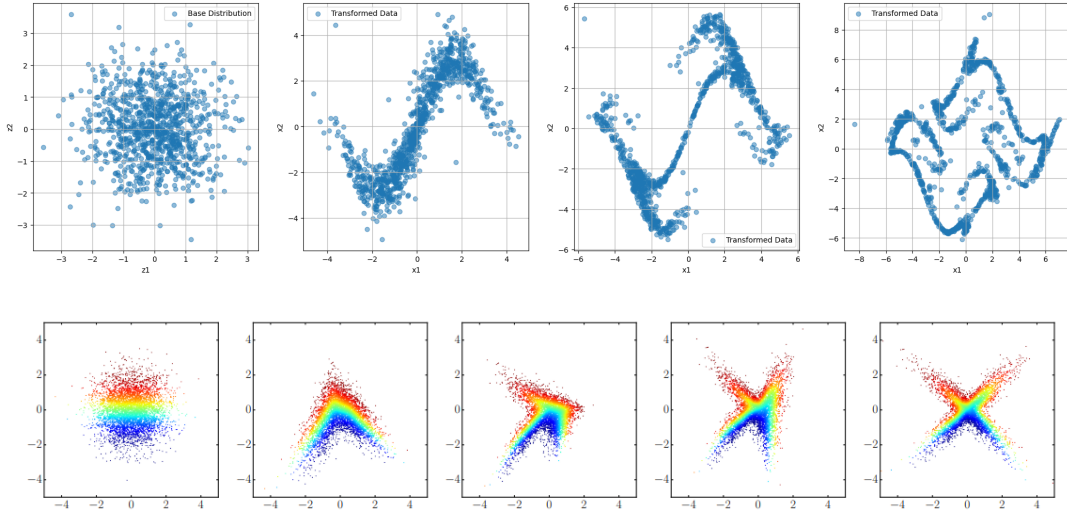
Figura 3.1: Esempi di composizione di trasformazioni di flow a partire da una distribuzione base gaussiana. In entrambi i casi si parte da campioni della gaussiana standard e si applica progressivamente una sequenza di trasformazioni T_k , ottenendo distribuzioni qualitativamente molto diverse dalla base.
