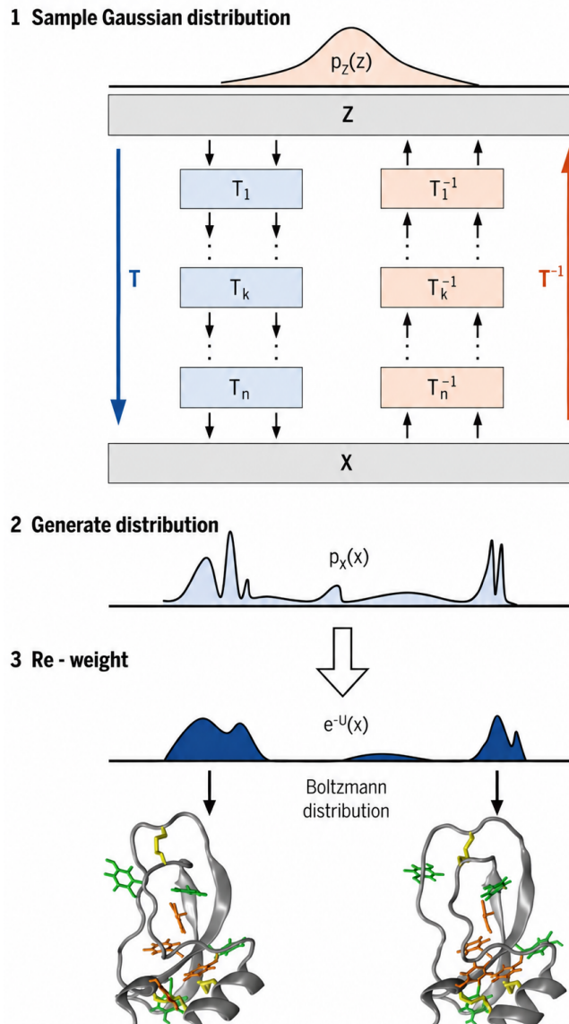
Figura 3.5: Boltzmann Generator: utilizza NF e re-weighting per campionare la distribuzione di Boltzmann. Nella figura si mostrano i passi di questo metodo e due configurazioni di una proteina rappresentati due modi distinti della distribuzione target.
