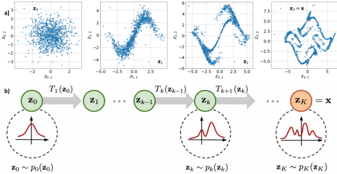
Figura 3.1: a : Esempio di composizione di trasformazioni per creare flow espressivo. Si campiona una distribuzione di base gaussiana e si applica progressivamente una sequenza di trasformazioni T_k , ottenendo distribuzioni qualitativamente molto diverse dalla base. b : Rappresentazione di un flow composto da K trasformazioni.
