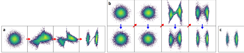
Figura 4.18: NF versus SNF per il potenziale doppio pozzo. Le frecce rosse indicano l'uso di una trasformazione deterministica, mentre le blu di una stocastica. a: 3 RealNVP blocks (2 layers each). b: Egualmente ma con 20 passi stocastici prima e dopo ogni RealNVP. c: Campioni dalla distribuzione target. Immagine tratta da [23].
