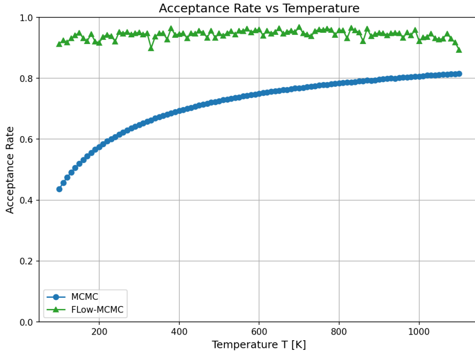
Figura 4.8: Tasso di accettazione medio di MCMC e Flow-MCMC in funzione della temperatura, a dimensione fissata D = 3 .
