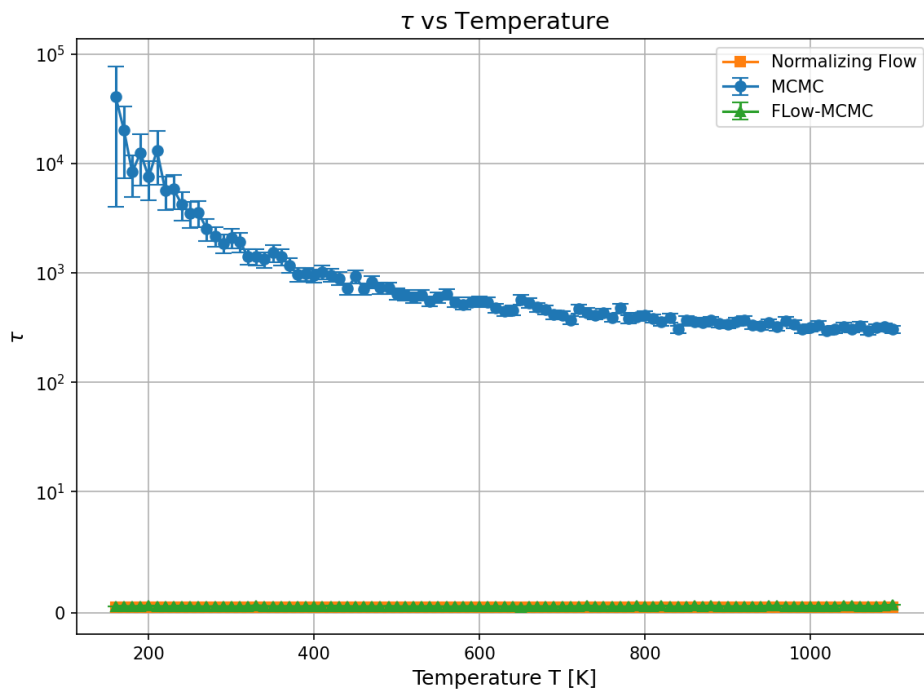
Figura 4.9: Si mostra \tau^{int} di x_1 per MCMC e Flow-MCMC e lo si confronta a \tau_{\text{eff}} = N/(2\text{ESS}) per NF. Tutti in funzione della temperatura e a dimensione fissata D = 3 .
