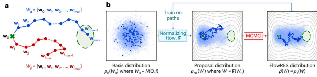
Figura 4.20: a: I percorsi di due particelle che partono dallo stesso punto w_0 (croce) e tentano la transizione verso la regione target (ellisse tratteggiata). Ogni percorso W è una sequenza di microstati. Il percorso W_\alpha (blu) effettua la transizione con successo, mentre W_\beta (rosso) non raggiunge il target. b: Schema del flusso di lavoro FlowRES, mostrato per il caso di particelle browniane passive che superano la barriera di un potenziale a doppio pozzo per raggiungere la regione target (ellisse tratteggiata). A sinistra: la traiettoria W_B (punti blu) viene campionata da una distribuzione gaussiana multivariata \rho_B(W_B) , con W_B \sim \mathcal{N}(0, I) . Al centro: un NF F trasforma W_B in un percorso proposto W' (linea blu) che verrà utilizzato come proposta di Metropolis-Hastings; la loro distribuzione \rho_{NF}(W') rappresenta dunque la distribuzione di proposta. A destra: i percorsi proposti vengono sottoposti a una fase di accettazione-rifiuto di Metropolis-Hastings, che convergerà alla distribuzione target dei cammini. La distribuzione FlowRES \hat{\rho}(W) addestra nuovamente F : ad ogni iterazione, la distribuzione proposta si adatta sempre meglio al target. Immagine tratta da [25].
