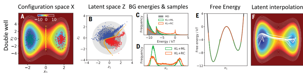
Figura 4.16: A: il potenziale con due traiettorie MD brevi (blu, rossa) che restano intrappolate ciascuna nel proprio stato metastabile. In arancione lo stato di transizione. B: Le traiettorie MD nello spazio latente. I due bacini blu e rosso diventano regioni distinte nella gaussiana latente. C: Distribuzione dell'energia potenziale campionata da MD (grigio) e BG (verde e arancione). D: Distribuzione dei campioni di BG rispetto alla coordinata lenta. E: Stime dell'energia libera ottenute dal flow dopo il re-weighting. F: Cammini generati interpolando linearmente nello spazio latente coppie (blu-rossa) di campioni MD. Immagine tratta da [21].
