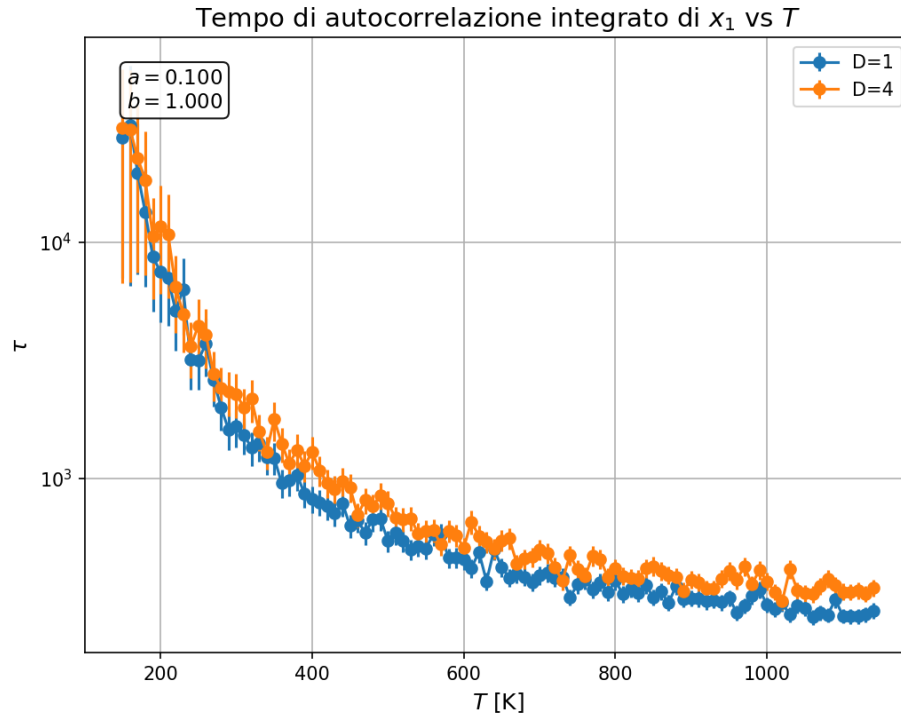
Figura 4.5: Tempo di autocorrelazione integrato \tau^{int} della coordinata lenta x_1 (in unità di passi di Metropolis) in funzione della temperatura, stimato con il metodo della finestra automatica di Sokal ( c = 5 ), per D = 1 e D = 4 .
