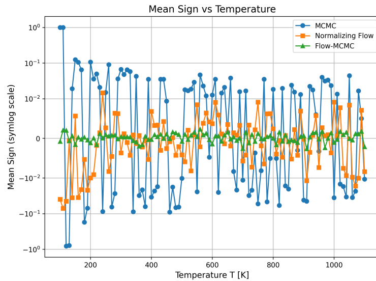
Figura 4.11: Segno medio \langle \text{sgn}(x_1) \rangle per MCMC, NF e Flow-MCMC in funzione della temperatura. L'asse verticale utilizza una scala logaritmica simmetrica, lineare per |\langle \text{sgn}(x_1) \rangle| < 10^{-2} . Il valore teorico atteso è nullo per ogni T .
