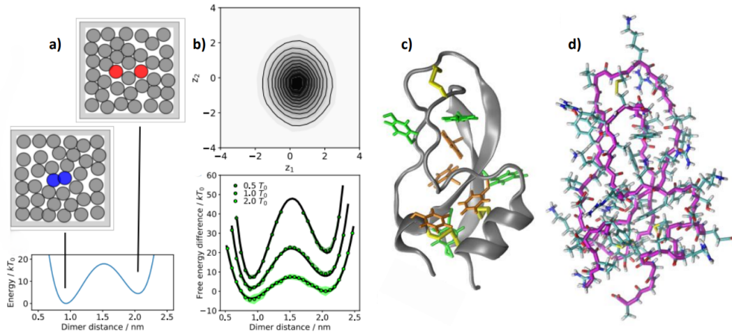
Figura 4.17: a: Configurazioni chiusa (blu) e aperta (rossa) del dimero e sotto il potenziale del dimero bistabile. b: Distribuzione dei dati delle simulazioni MD nelle coordinate dello spazio latente z_1, z_2 . Sotto le differenze di energia libera in funzione della distanza del dimero e della temperatura campionate tramite BG. c: Struttura cristallografica a raggi X di BPTI. d: Campione generato tramite BG di tutti gli 892 atomi della proteina BPTI, analogo alla struttura a raggi X. Immagini tratte da [21].
