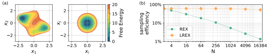
Figura 4.19: a: Potenziale doppio pozzo N -dimensionale usato come sistema di test, con le prime due coordinate bimodali e le restanti armoniche. b: Efficienza di campionamento di REX (verde) e LREX (arancione) in funzione della dimensionalità N , in scala log-log: REX diminuisce all'aumentare di N , LREX resta pressoché costante. Immagine tratta da [24].
