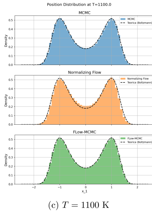
Figura 4.14: Istogramma, normalizzato a densità di probabilità, della coordinata x_1 campionata da MCMC, NF e Flow-MCMC, confrontato con la distribuzione di Boltzmann marginale ottenuta per integrazione numerica (linea tratteggiata), a tre diverse temperature, D = 3 .
