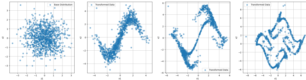
Figura 3.3: Esempio di espressività di un flow composto. La prima immagine mostra i campioni della distribuzione base gaussiana, mentre le successive mostrano la distribuzione ottenuta applicando progressivamente la trasformazione T_k : dopo 2, 4 e 8 trasformazioni consecutive. Si può osservare come, grazie all'elevata espressività delle singole trasformazioni T_k , già con un numero limitato di trasformazioni sia possibile ottenere distribuzioni qualitativamente molto diverse dalla distribuzione base.
