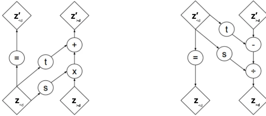
Figura 3.5: Rappresentazione grafica di un T_k per una Real NVP. Possiamo vedere la suddivisione del vettore \mathbf{z} e il calcolo di \mathbf{s} e \mathbf{t} rispettivamente i fattori di scaling e translation. A sinistra la trasformazione e a destra la sua inversa.
