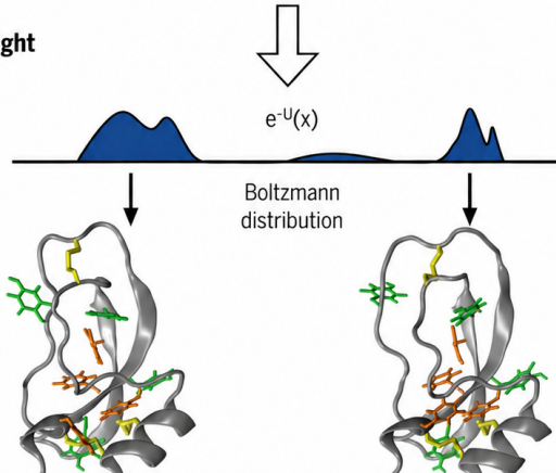
Figura 3.5: Boltzmann Generator: utilizza NF e re-weighting per campionare la distribuzione di Boltzmann. Nella figura si mostrano i passi di questo metodo e due configurazioni di una proteina rappresentati due modi distinti della distribuzione target.
