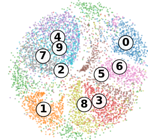
EntroPath (sil=0.096)
