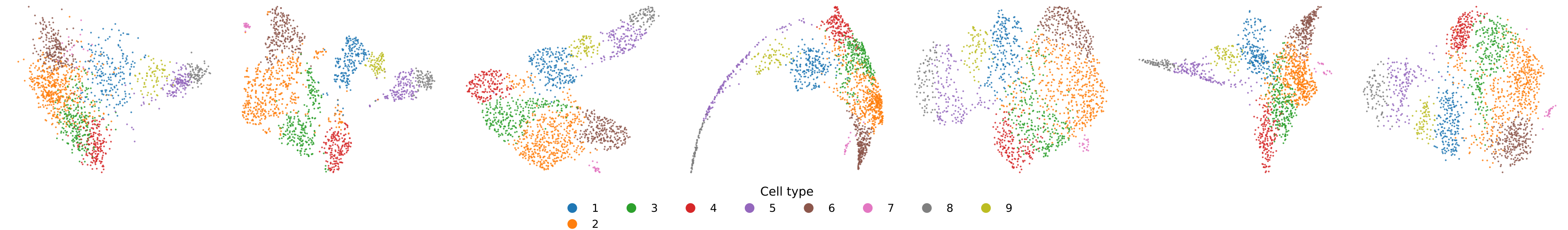
PCA
