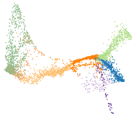
DTNE
