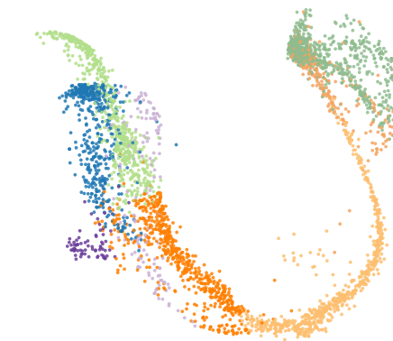
EntroPath
