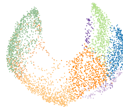
HeatGeo
