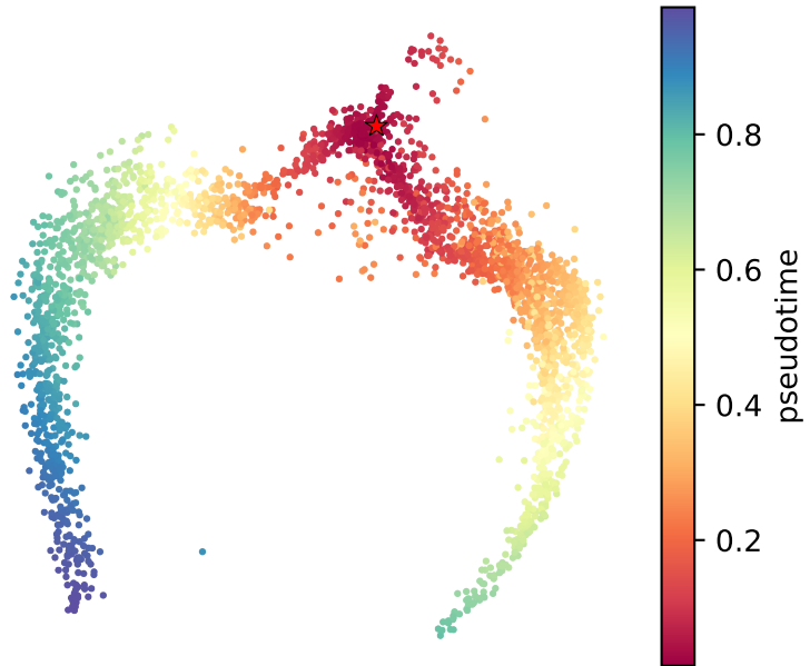
EntroPath
